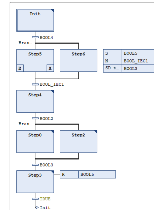
SFC (последовательная функциональная диаграмма)
