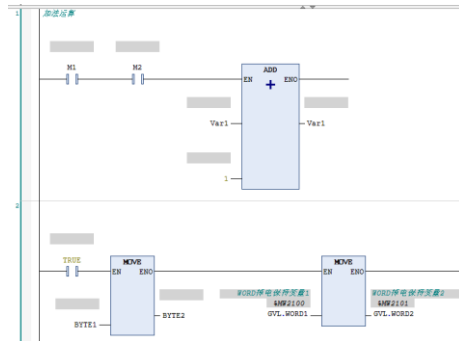
LD (релейно-контактная схема)
