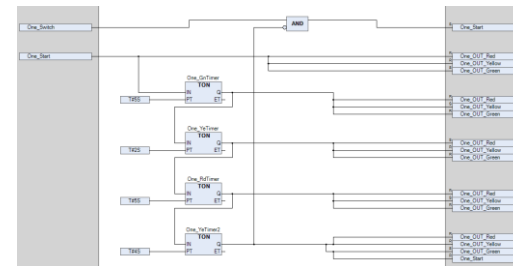
CFC (непрерывная функциональная диаграмма)
